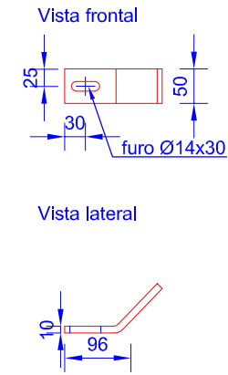
6 Br50x10 (Esc. 1/10)
