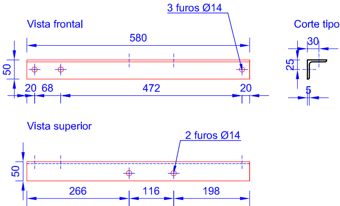
8b L50x50x5 (Esc. 1/10)
