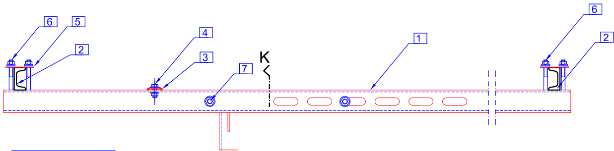
Vista superior
