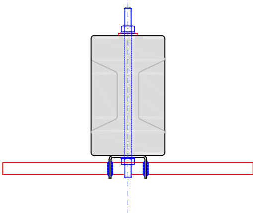
Corte K
