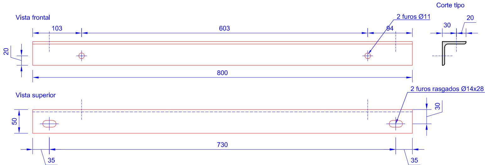
1e L50x50x5 (Esc. 1/5)
