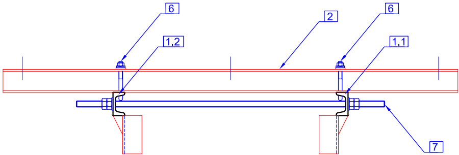
Corte K
