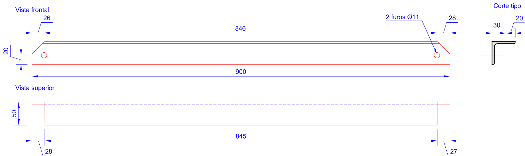
2e L50x50x5 (Esc. 1/5)
