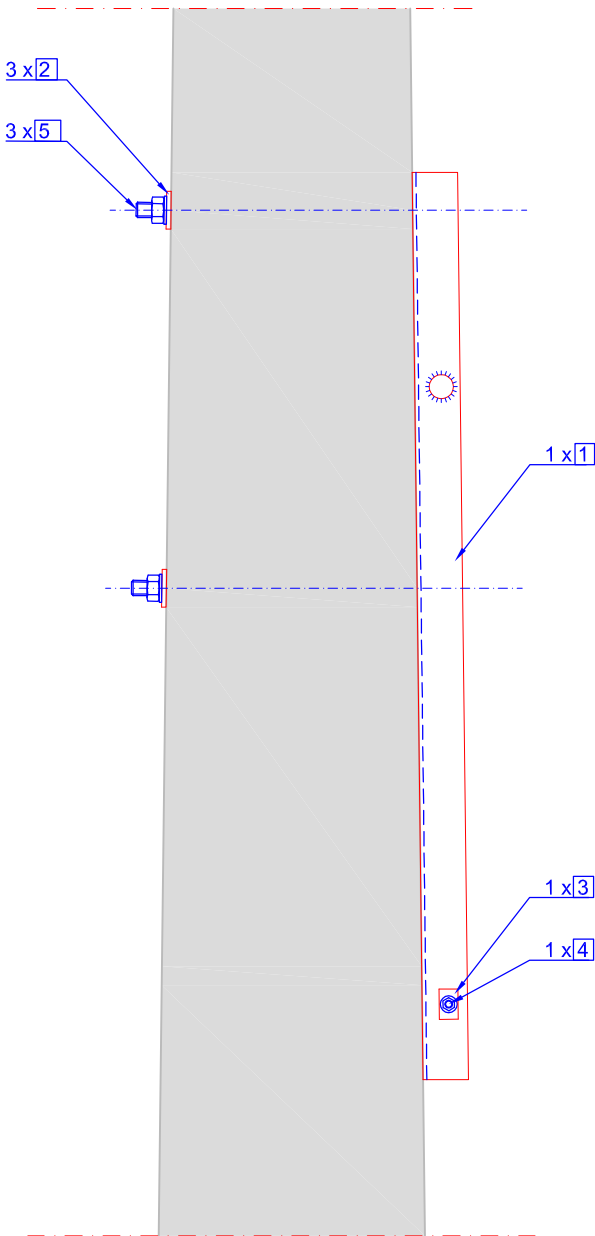
Vista lateral
