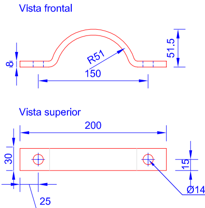
10 P12-360(50)+P(2)+AP(2) (Esc. 1/2)
