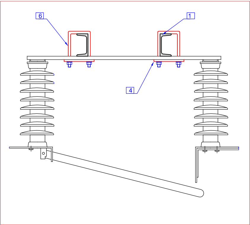
Corte K Esc. 1/10
