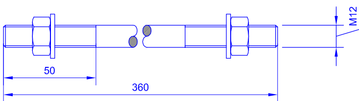
10 P12-360(50)+P(2)+AP(2) (Esc. 1/2)
