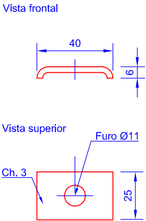
18 FLT40x25x3 (Esc. 1/2)
